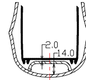
下管走线空间图
