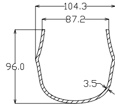
下管开口截面图
