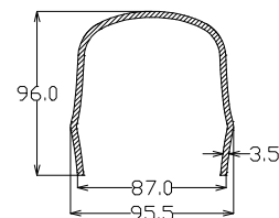
下管开口截面图
